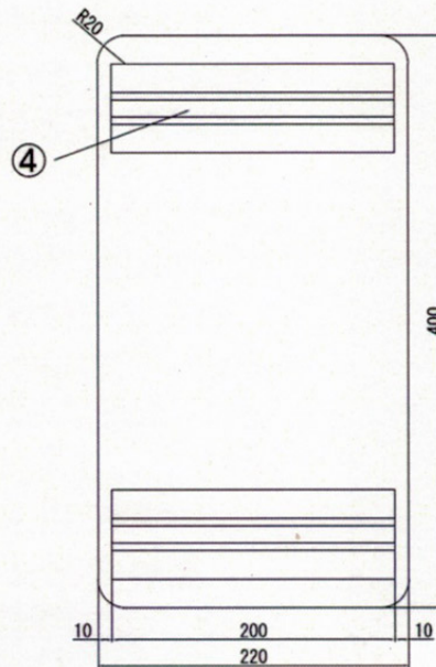
裏面図
